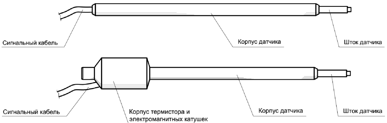
Рис. 2.1. Общий вид струнных датчиков перемещения SJ-3000, SJ-3010, SJ-3015
